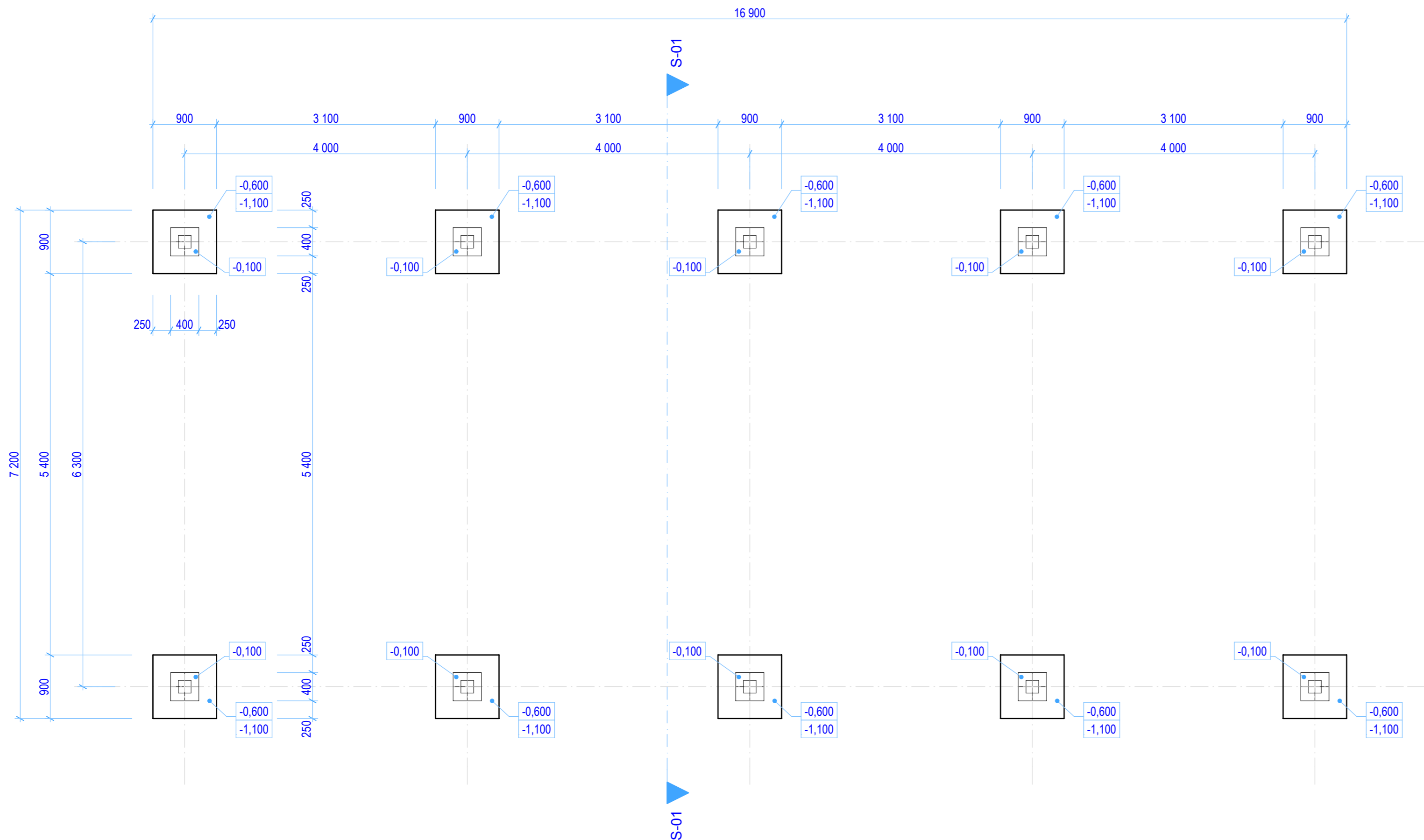
PÔDORYS ZÁKLADOV PAVILÓNU M=1:50
